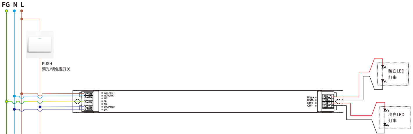
接线图
